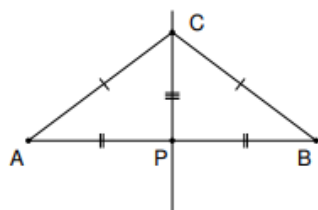
Slika 3: simetrala dužine
