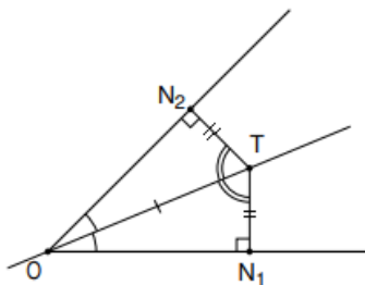
Slika 4: simetrala kuta
